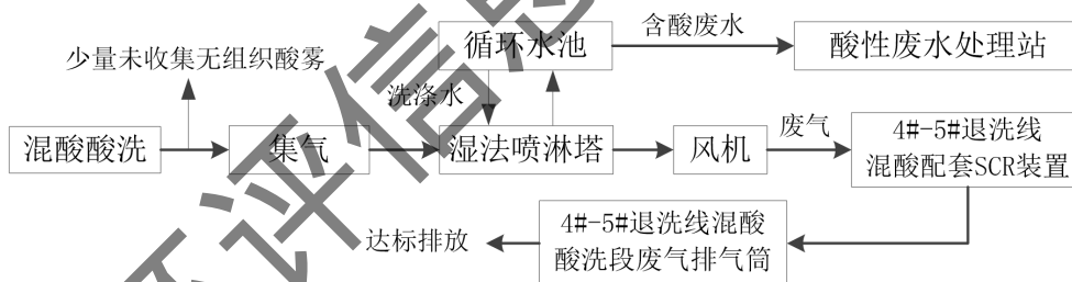
图 4.5.4 混酸酸洗废气处理工艺流程示意图
